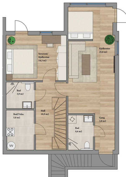
Caroline Øverlands vei 49A - underetasje Skala 1:50
